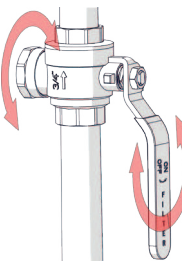
Magnetfilter-Kugelventil
