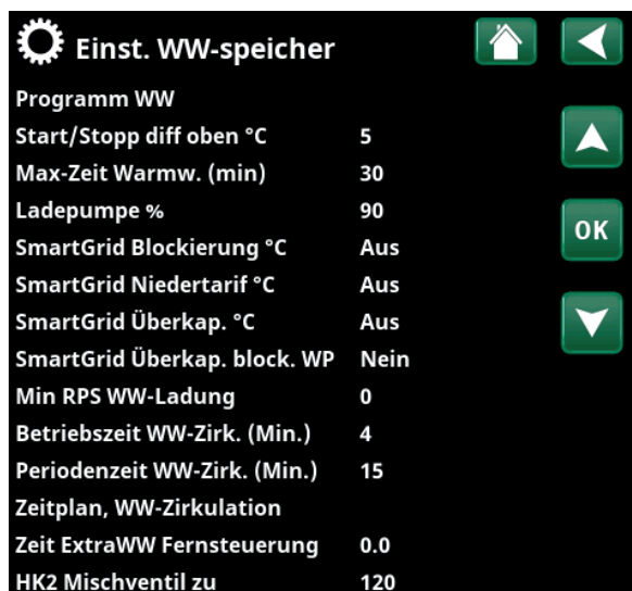
Ausschnitt aus dem Menü „Erweitert/Einstellungen/WW-Speicher“.
