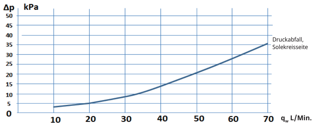
CTC GSi 616
