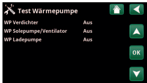
Menü: „Erweitert/Service/Funktionstest/Wärmepumpe“.
