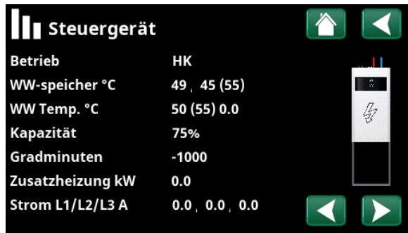
„Menü Betriebsdaten/Steuergerät“. Die Pfeile anklicken oder seitlich wischen, um zum Menü „Betriebsdaten/Wärmepumpe“ zu wechseln.
