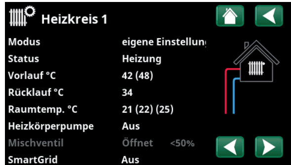
Das Menü zeigt detaillierte Betriebsdaten des ausgewählten Heizkreises an. Zur Anzeige festgelegter Heizkreise die Pfeiltasten anklicken oder seitlich wischen.
