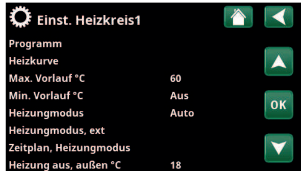
Ausschnitt aus dem Menü „Erweitert/Einstellungen/Heizkreis/Heizkreis 1“.
