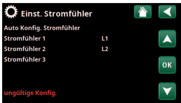
Menü: „Erweitert/Einstellungen/Stromfühler“.
